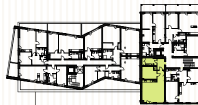
Půdorys podlaží
