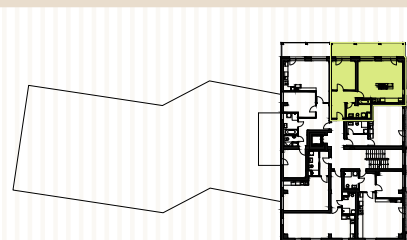
Půdorys podlaží
